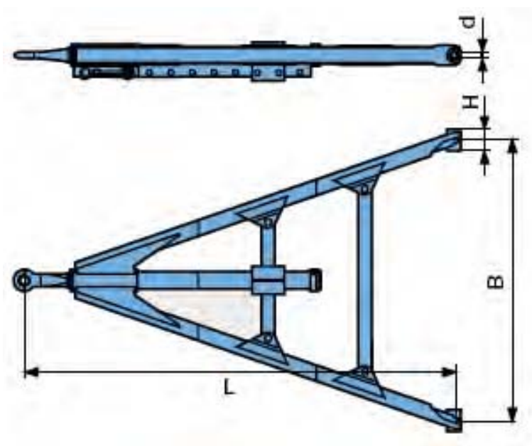
Bild 4 Zuggabel längenverstellbar
