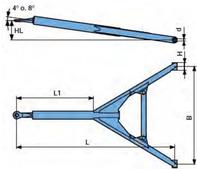
Bild 5 Mittelholmszuggabel, gerade oder geneigte Zugöse
