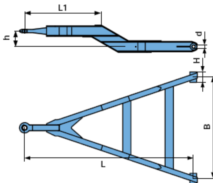
Bild 6 Zuggabel gekröpft
