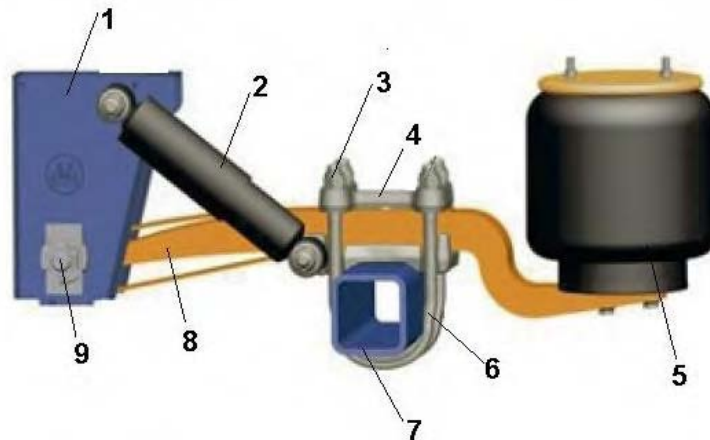
Bild 11 Luftfederung
